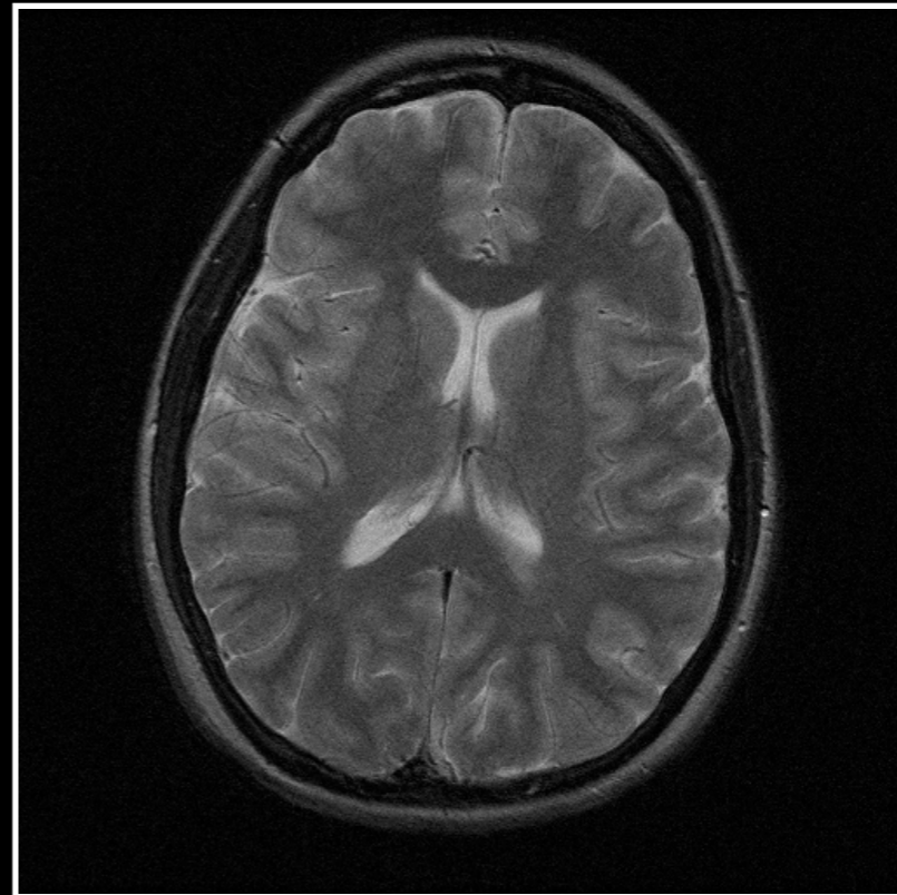
POCS
